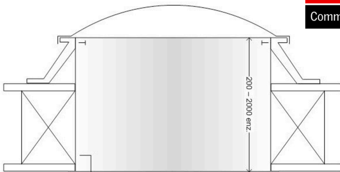
Doorsnede A Cross section A Querschnitt A
